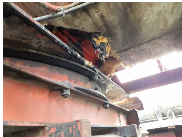
Beschädigung 12: Tankfahrzeug: Tankkammer (Isolierung u. Tank Kostenausweitung möglich) - undicht - instandsetzen
