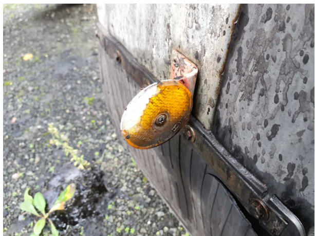
Beschädigung 2: Aufbau: Aufbau (MarkierungsReflektor vorn rechts) - gebrochen / gerissen - erneuern
