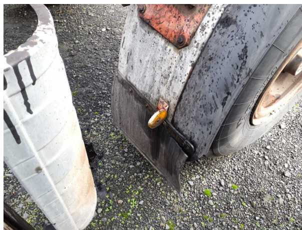
Beschädigung 2: Aufbau: Aufbau (MarkierungsReflektor vorn rechts) - gebrochen / gerissen - erneuern
