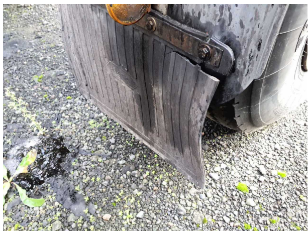
Beschädigung 1: Kotflügel rechts: Kotflügel rechts (Spritzschutz) - gebrochen / gerissen - erneuern
