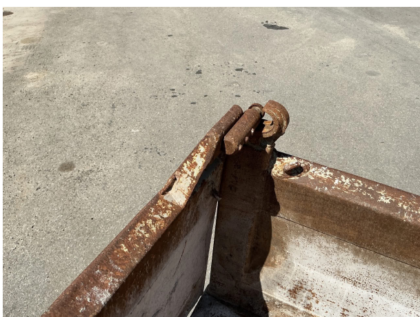
Beschädigung 6: Dreiseitenkipper: Bordwand hinten - verformt - erneuern
