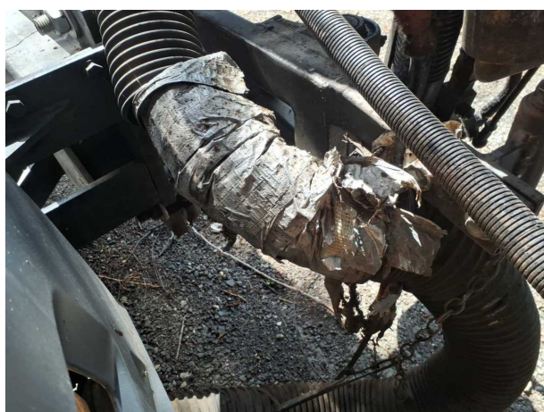
Beschädigung 3: Anbauteil rechts: Anbauteil (Frontarbeitsarm Schtzhülle) - beschädigt - erneuern
