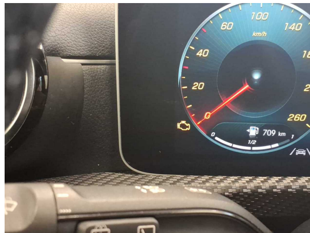
Beschädigung 1: Instrumententafel: Kontrollleuchte (Sporadisch, glühkerzen fehler) - leuchtet - Diagnose
