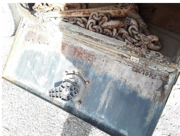
Beschädigung 4: Rahmen: Rahmen (Staukasten durchgerostet) - erneuern
