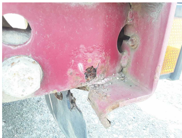
Beschädigung 3: Rahmen: Unterfahrschutz hinten - verformt - instandsetzen und lackieren
