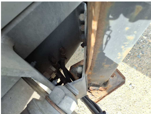
Beschädigung 5: Sonstiges: Fahrzeug (Stützbein , und Korrosion) - verformt - erneuern
