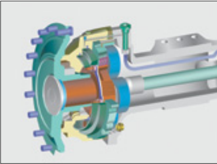
Diferencial ZF de deslizamiento limitado Los ejes poseen diferenciales de desplazamiento limitado en las partes delantera y trasera. Esto garantiza, de manera automática, el máximo esfuerzo de tracción y un desplazamiento cómodo sobre terrenos blandos y lodosos. También reduce el riesgo de patinar y, al mismo tiempo, evita el desgaste excesivo de los neumáticos. Los discos de freno se han reubicado a la parte trasera del engranaje de reducción, donde la velocidad de rotación es menor. Como resultado, quedan expuestos a menos rpm, disminuye la generación de calor y su vida útil aumenta en gran medida.
