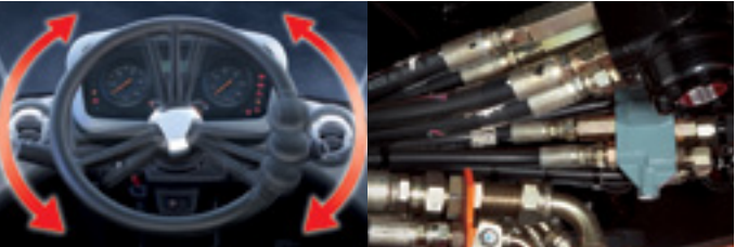
Dirección hidráulica El nuevo diseño del sistema de dirección garantiza un control uniforme aun con bajas revoluciones del motor.
