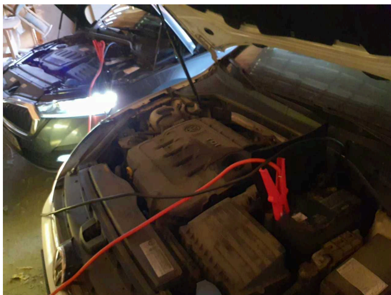
Beschädigung #6: elektrisches System: Batterie - defekt - erneuern
